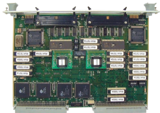
マルチDSPボード
