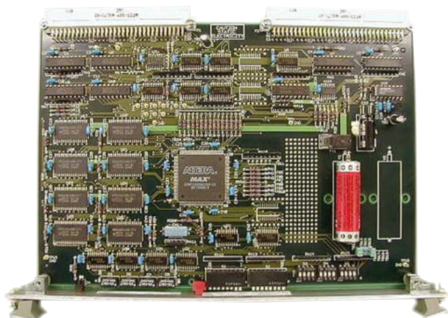
観測レーダー受信インターフェイス
