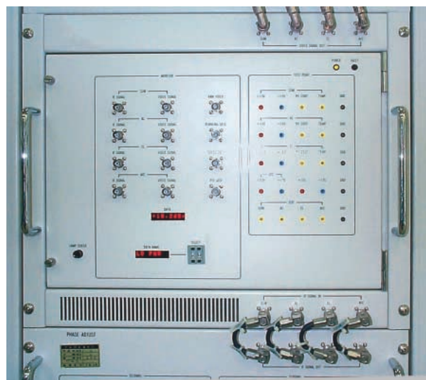
観測レーダー復調ユニット
