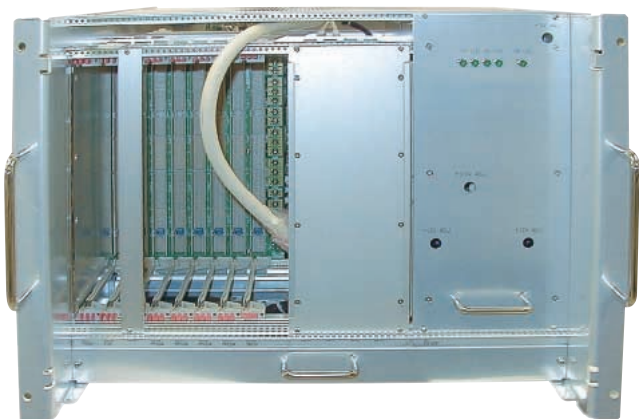
気象観測信号処理装置
