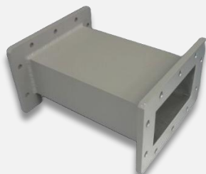
WRJ-2規格ストレート管
