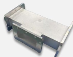
H面T分岐導波管
